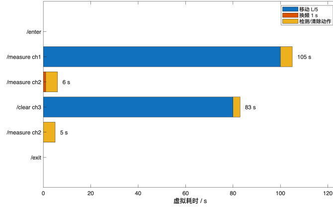
图 3 附件计时示例的逐动作构成。移动项为距离除以 5 m/s，标题数字为该步合计。
