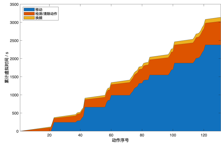
图 11 一局全向演练（BBM9-HZG2-77N5-NKKC，10 个源）的累计虚拟时间构成。该局为演练案例，不计入正式测试结果。
