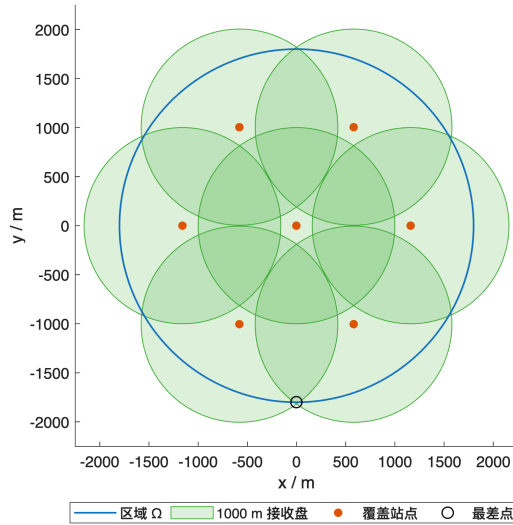
图 6 七点全向覆盖构造。站点取自配置参数 a = 1159.7 \text{ m} , 圆圈为 1000 \text{ m} 接收盘, 最差点位于 (0, -1825) 附近, 最坏距离 \leq 984.539 \text{ m} 。
