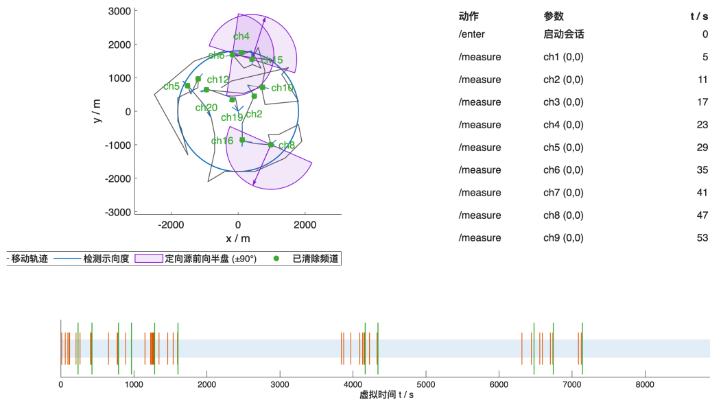
图 9 含定向源演练局（GHSN-M38E-74GD-YLUD）的运行回放，紫色半盘为定向源的前向可见区域。该局为演练案例，非正式测试记录。
