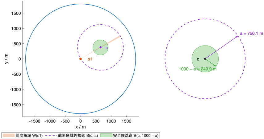
图 5 第二点解析候选区域。左图为首次截断角域 S 、其最小包围圆 \overline{B}(c, a) 与保证接收的候选盘 \overline{B}(c, 1000 - a) ；右图为半径分解， a = 1500/(2 \cos \delta) 。取 \delta = 1^\circ 时 a \approx 750.114 \text{ m} 、 1000 - a \approx 249.886 \text{ m} ，与表 3 一致。
