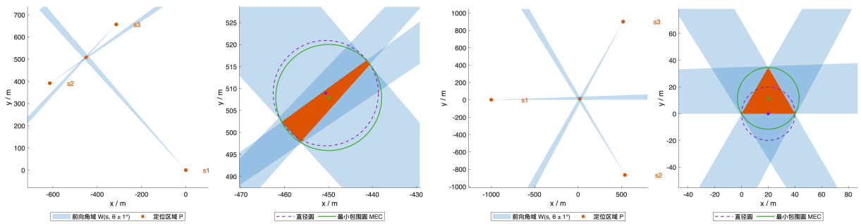
图 4 问题一的两组几何。(a) 三点交会算例：定位区域及其直径圆与最小包围圆，观测取自官方演练案例 U5ZW-P9KN-TCAG-R7ST 的频道 9，几何量由生产求解器 mcm26b.geometry.solve 现算；(b) 等边三角形解析反例，虚线直径圆 r = 20 m 不覆盖顶点 C ，实线最小包围圆 \rho = 40/\sqrt{3} \approx 23.094 m 覆盖全部顶点，不是模拟器观测。
