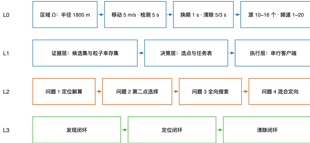
图 1 四问共用的模型链路：题面抽象（L0）、在线三层（L1）、四问主线（L2）与发现、定位、清除三个闭环（L3）。
