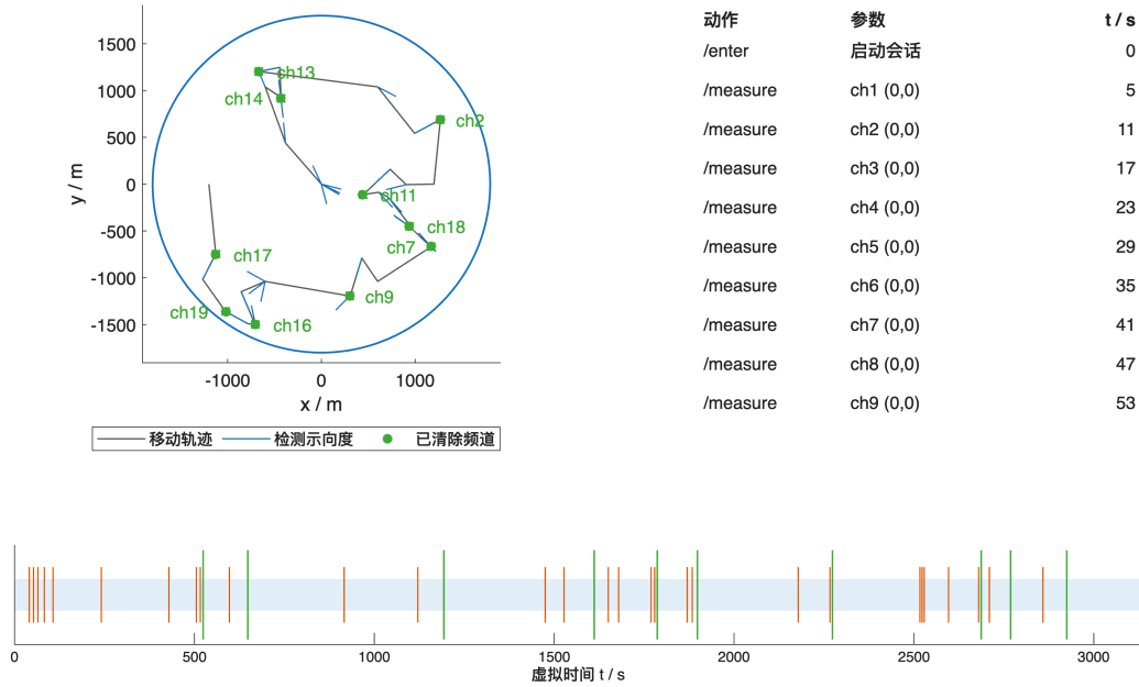
图 7 全向源演练局（BBM9-HZG2-77N5-NKKC）的运行回放。该局为演练案例，非正式测试记录。
