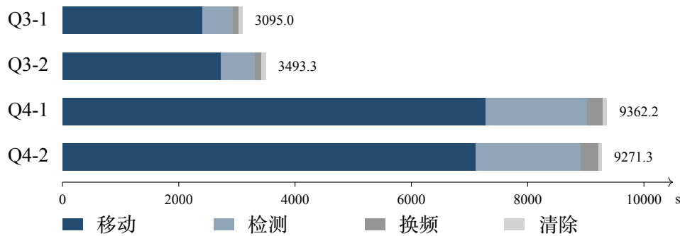
图 10 四次正式测试的累计虚拟耗时。移动项由总时间扣除官方动作计数对应耗时反推。
