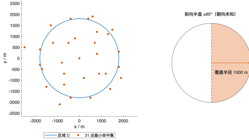
图 8 31 点最小命中集的几何分布（左）与定向源的前向半盘语义（右）。站点取自计划文件，部分站点位于 \Omega 之外，用于接收向外发射的边界源；离散校验不等同于连续覆盖证明。
