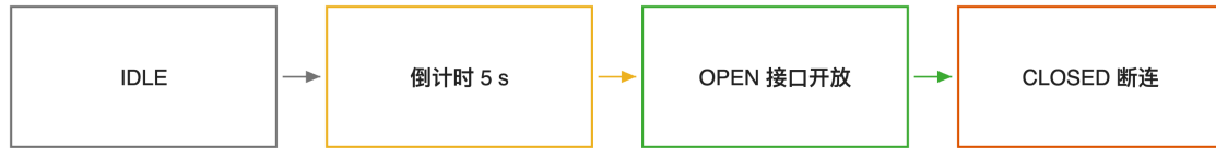
图 2 会话状态机。进入后经 5 s 倒计时接口开放，主动退出或断连后进入关闭状态。
